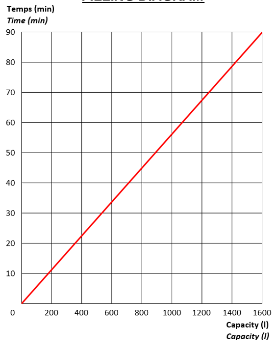
COURBE DE REMPLISSAGE FILLING DIAGRAM
